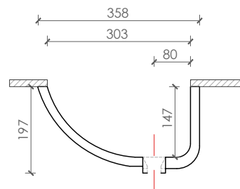
Alzado Lateral
